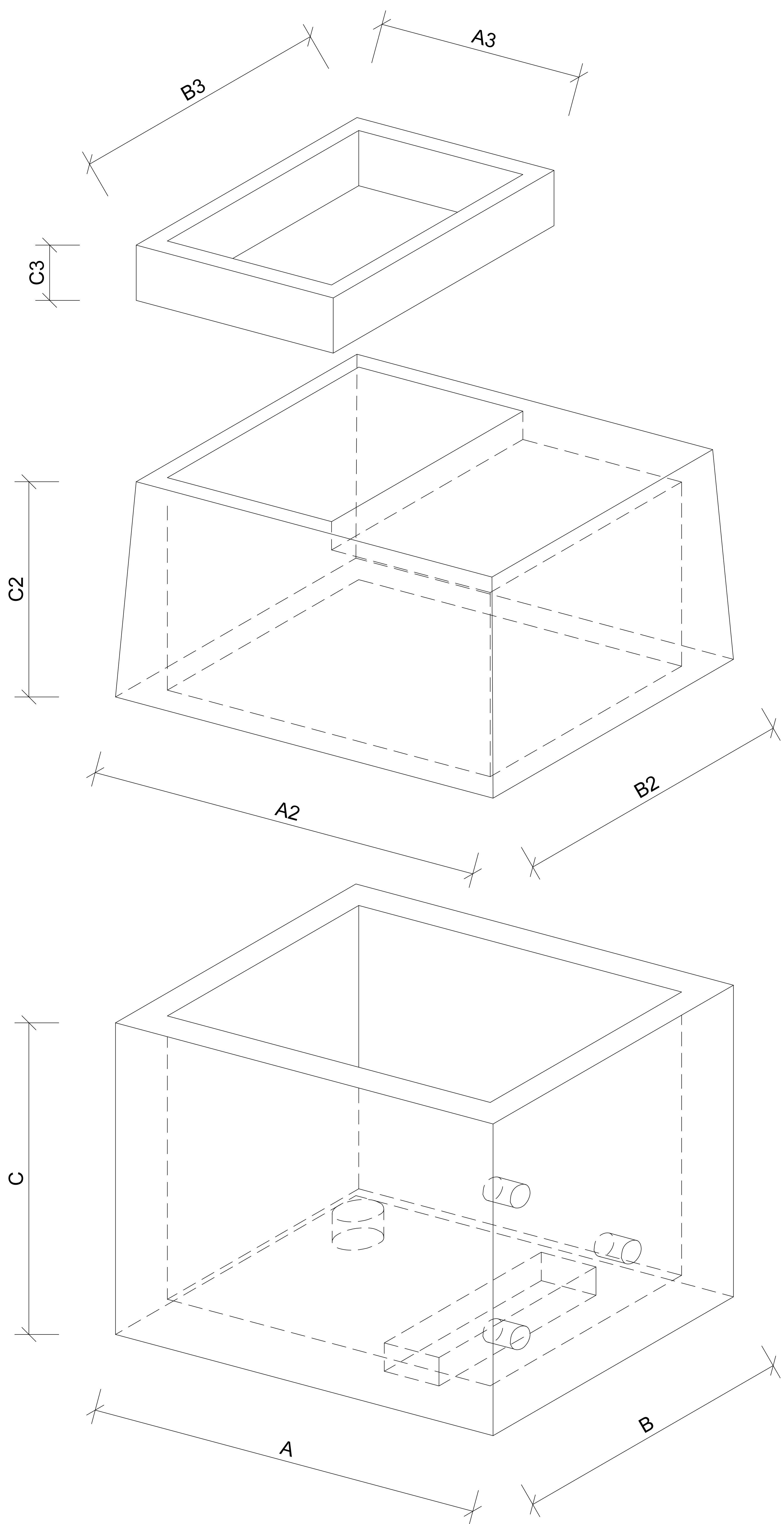
ZASNEŽOVACIA ŠACHTA
